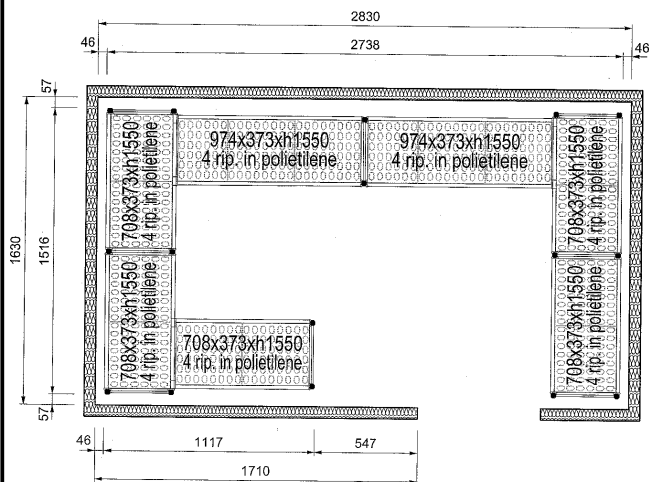
Boven aanzicht
